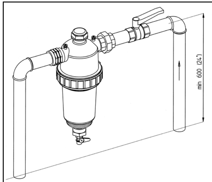
Fig. 1: Installation en ligne
