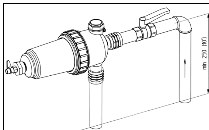
Fig. 2: Installation en angle 90°
