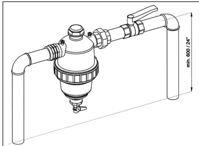
Fig. 1: Installation en ligne
