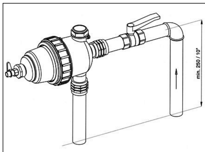
Fig. 2: Installation en angle 90°
